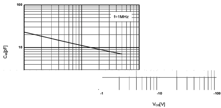
C_{ob} - V_{CE}
