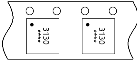
编带示意图
