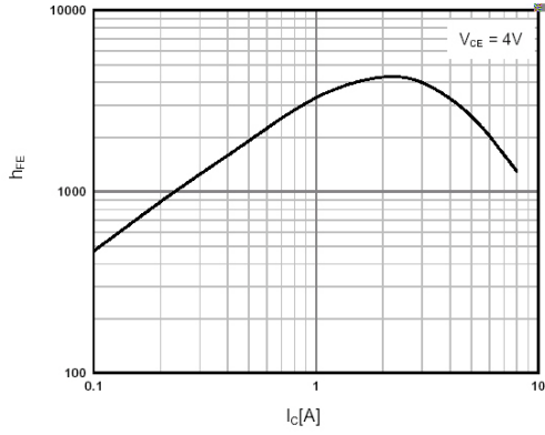
hFE - IC
